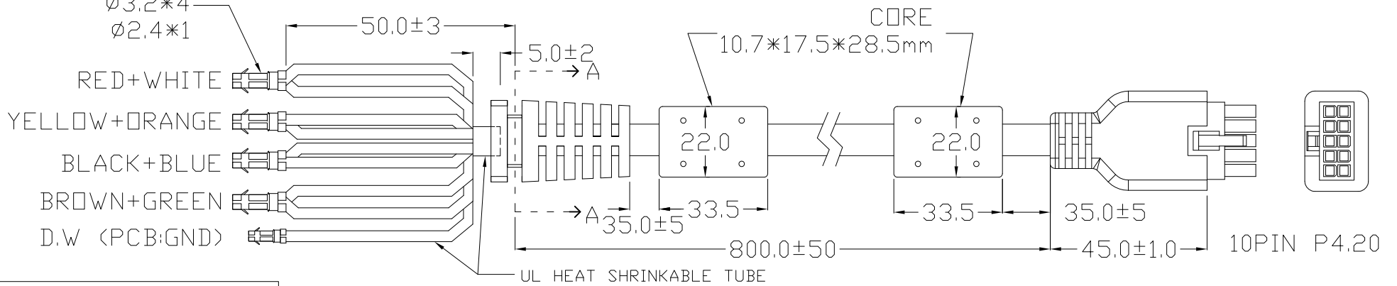
FRONT VIEW 10P DIN
