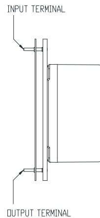
MOUNTING (D)
