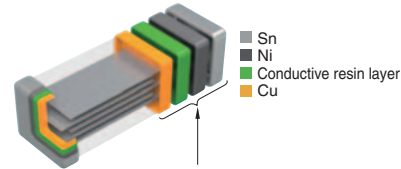
树脂电极品（以往款式）
