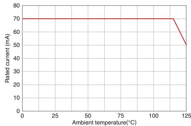
额定值降低
